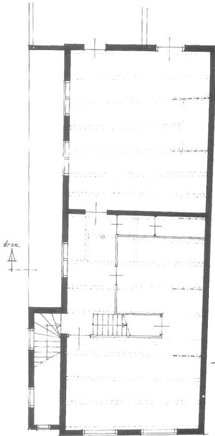
17. Plattegrond van de eerste verdieping na de restauratie.
