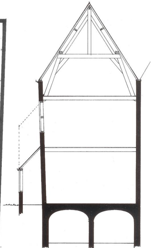
18. Doorsnede na de restauratie. Vorm van de kelders bij benadering.
